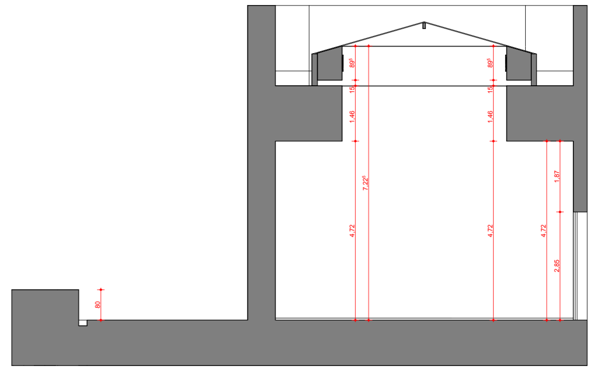
SECTIUNEA J-J
