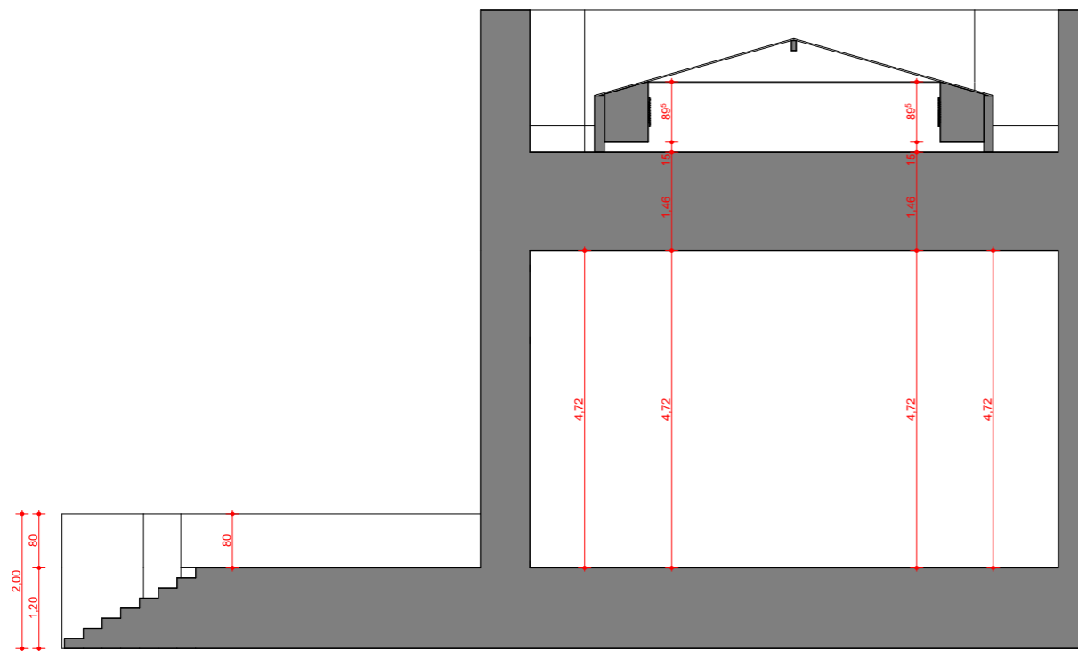
SECTIUNEA I-I
