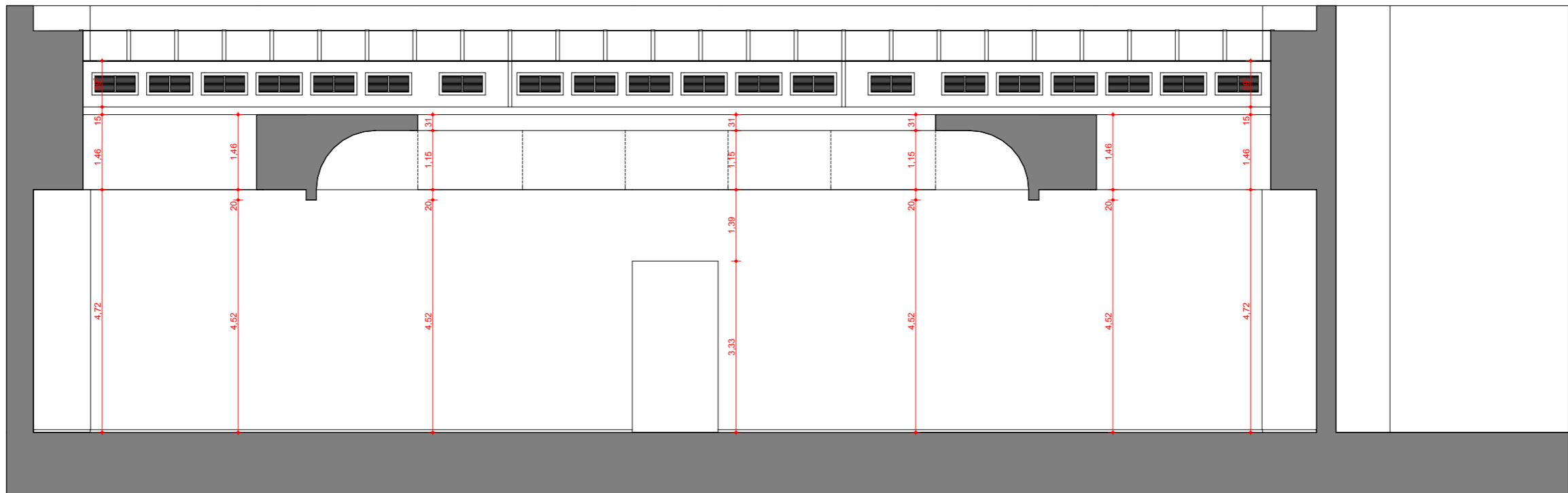
SECTIUNEA D-D
